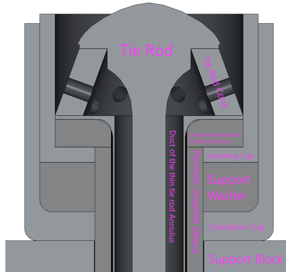
(d) Support block hardware detail
